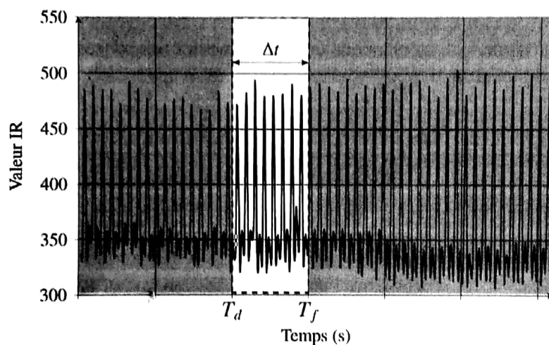
Figure 4 - Fenêtrage du signal
