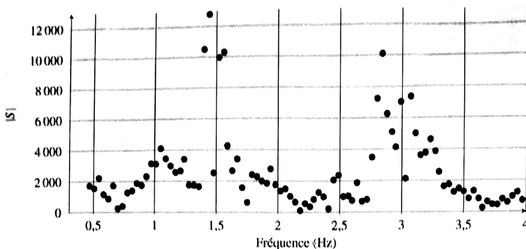
Figure 3 - Spectre issu de la TFD pour f \in [0,2 \text{ Hz}, 4 \text{ Hz}]
