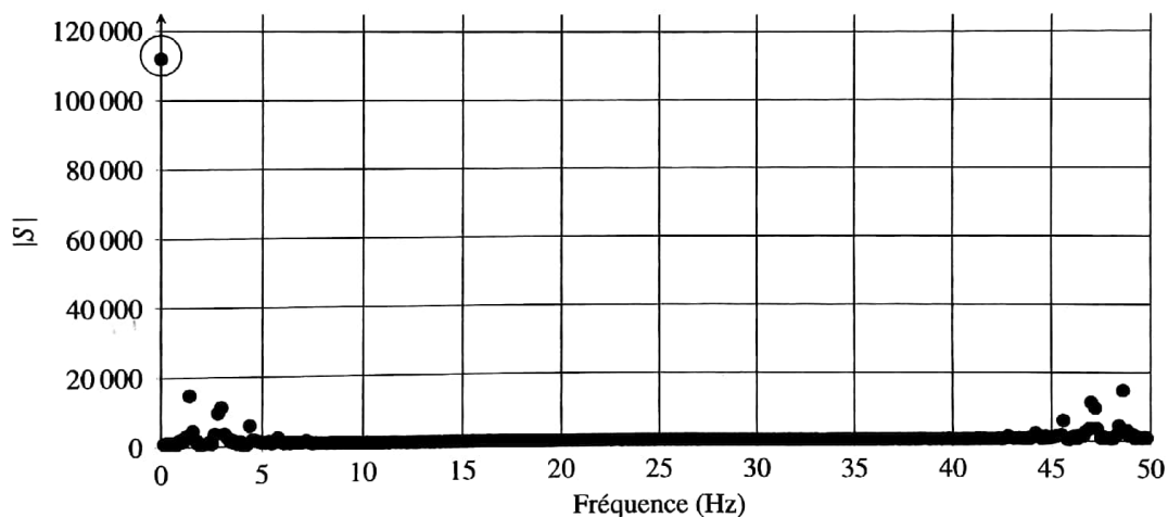
Figure 2 - Spectre après application de la TFD
