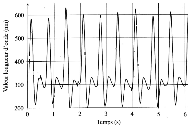
Figure 1 - Mesure PPG : tracé de la liste signal en fonction de la liste temps
