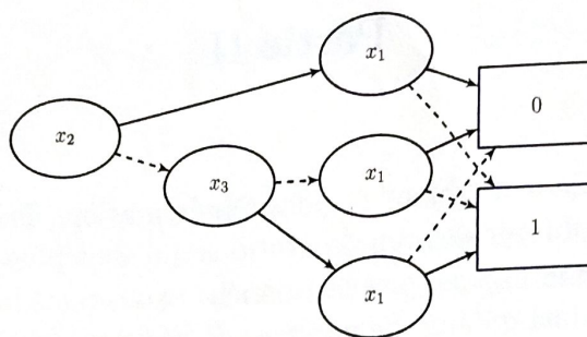
FIGURE 1 – Un ADBO où les arêtes avec étiquette 0 sont représentées en pointillés
