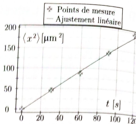
FIGURE 2 – Diffusion de grains
