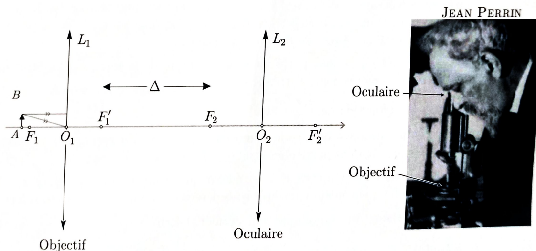
FIGURE 3 – Schéma d'un microscope (à gauche) – JEAN PERRIN observant les grains (à droite)
