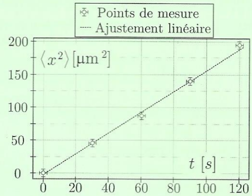
FIGURE 2 – Diffusion de grains
