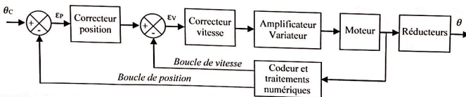
Figure 13 - Structure de l'asservissement d'un axe
