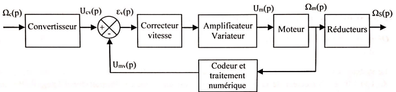
Figure 14 - Asservissement en vitesse d'un axe
