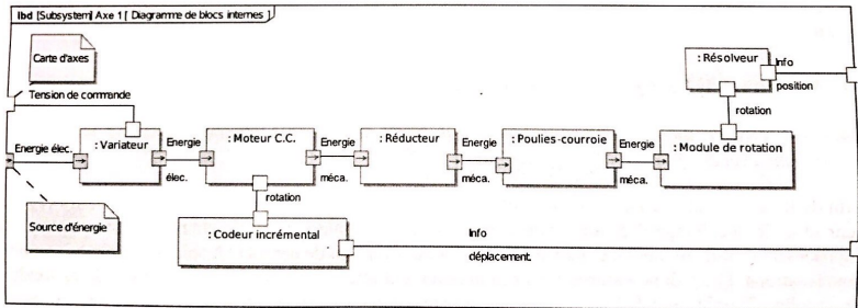
Figure 4 - Diagramme de blocs internes de l'axe 1
