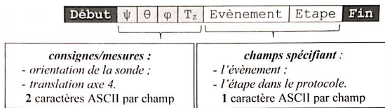
Figure 22 - Structure des paquets de données échangés
