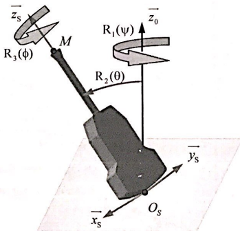
Figure 7 - Repère lié à la sonde et rotations
