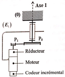
Figure 3 - Chaîne cinématique associée à l'axe 1
