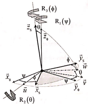
Figure 8 - Angles d'Euler
