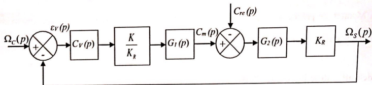
Figure 15 - Schéma-bloc équivalent pour la boucle de vitesse
