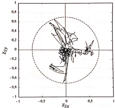
Figure 19 - Évolution de l'inclinaison de la sonde lors d'un examen d'échographie classique
