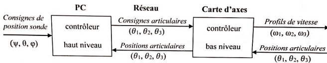
Figure 12 - Principe de la commande du robot porte-sonde
