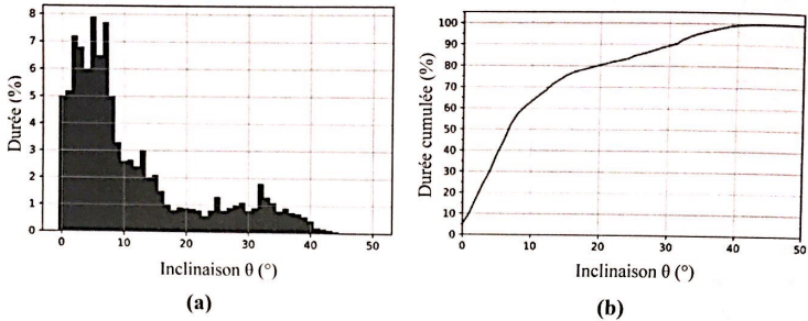
Figure 20 - Histogramme (a) et diagramme des durées cumulées (b) générés par le code Python
