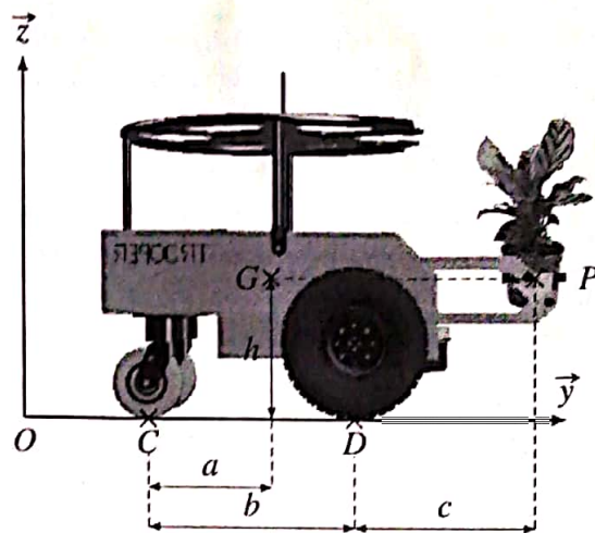
Figure 14 - Paramétrage pour l'étude du basculement
