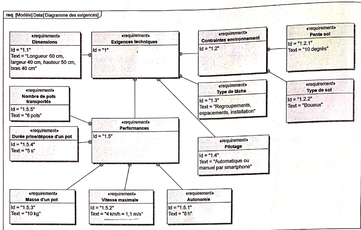
Figure 4 - Diagramme des exigences du robot Trooper
