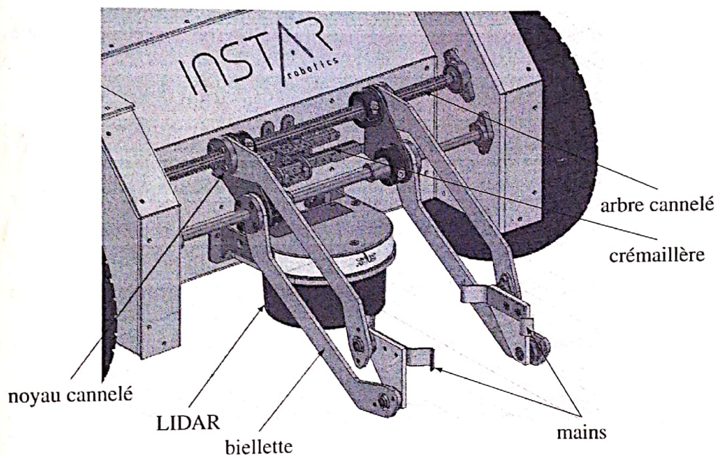
Figure 10 - Description du mouvement bras
