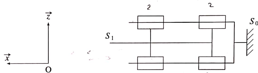
Figure 12 - Modélisation simplifiée des liaisons entre la crémaillère et le châssis
