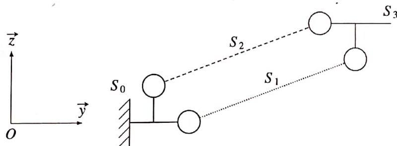
Figure 13 - Modélisation simplifiée du mécanisme d'élévation
