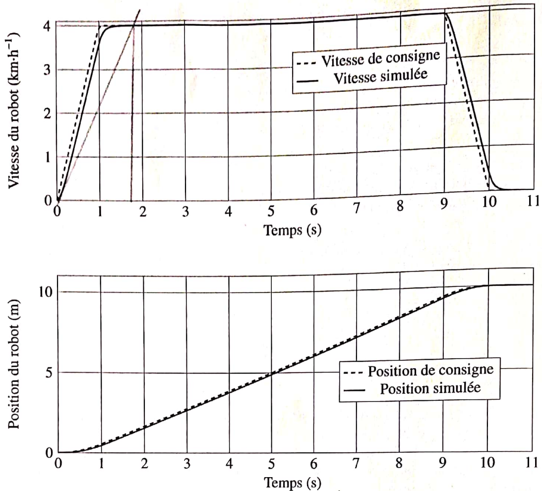
Figure 5 - Simulation du déplacement du robot en réponse à une consigne en trapèze
