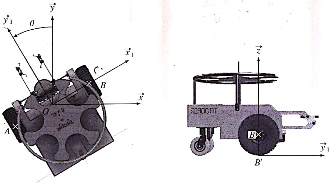
Figure 8 - Paramétrage du robot en virage
