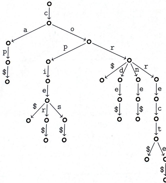
FIGURE 1 – Exemple de trie de taille 28 contenant 9 mots.
