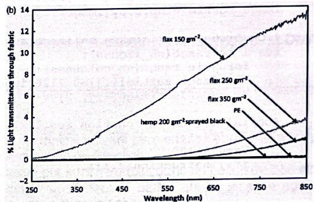
(b) Transmittance de la fibre de lin
