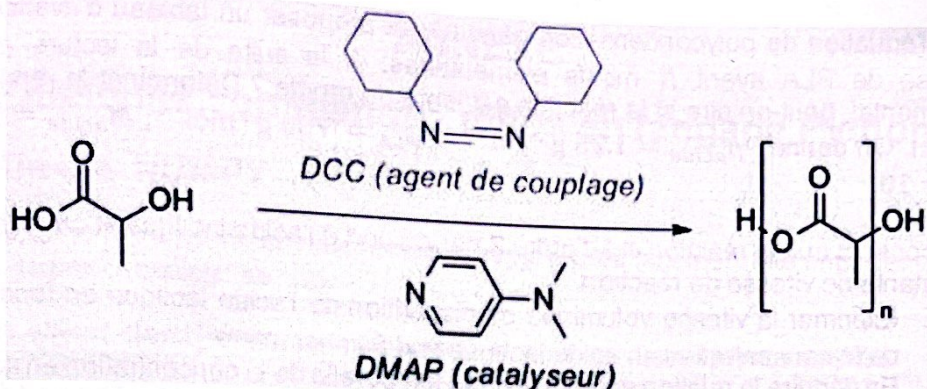
Figure 10 - Synthèse du PLA par polymérisation
