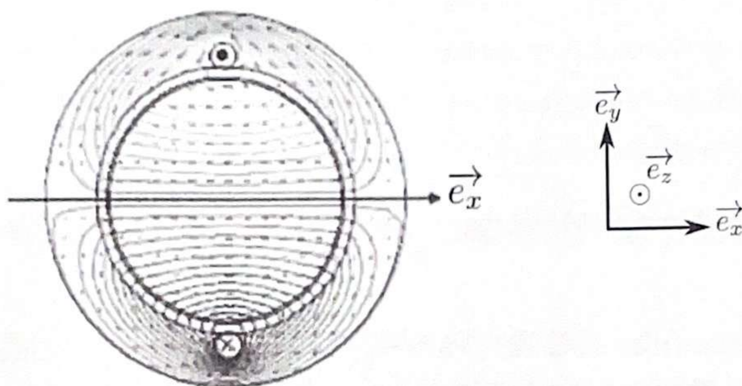
Figure 8 - Champ magnétique créé par la spire centrale de l'enroulement S_1 du stator.
