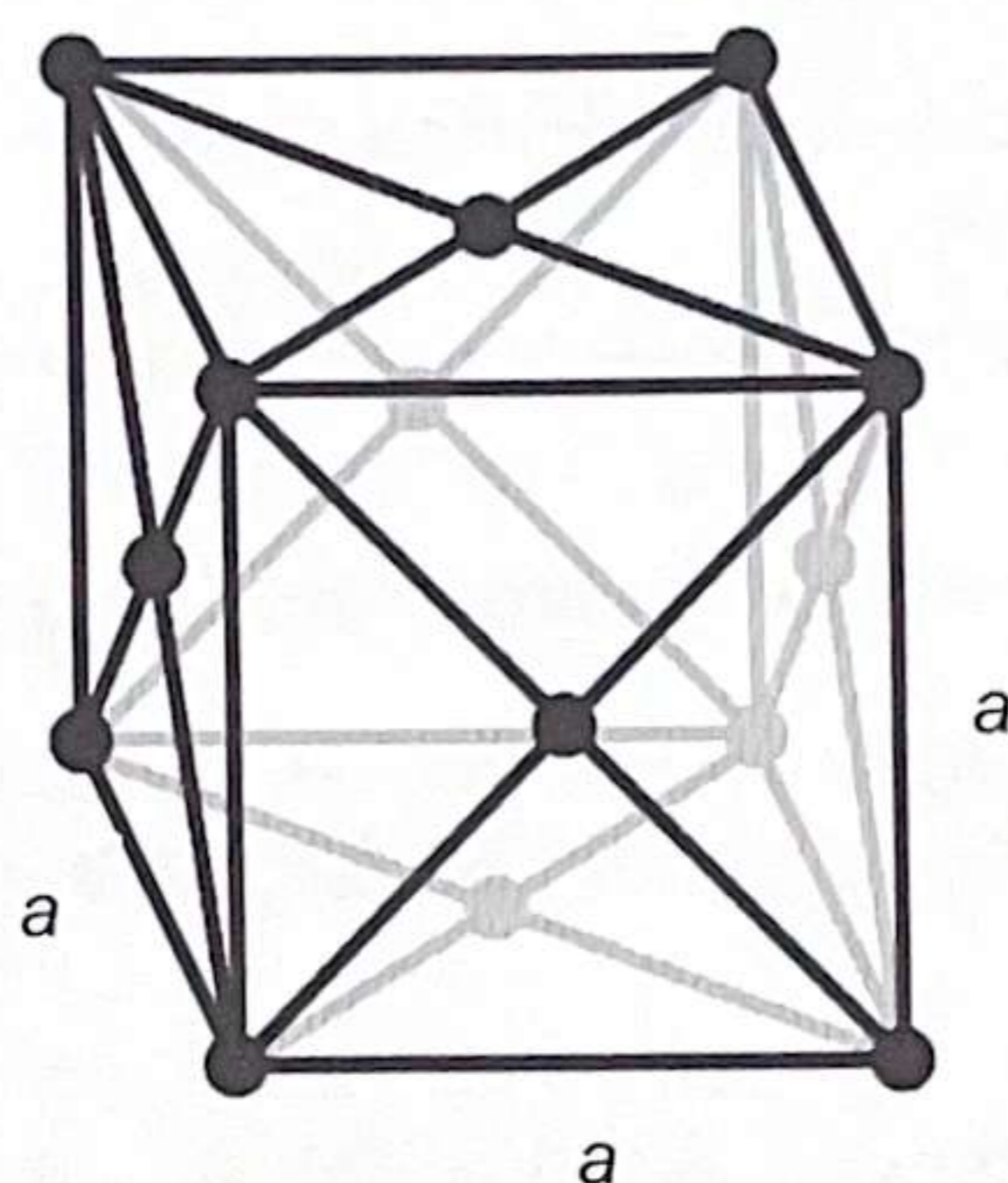
Figure 3 - Structure de type cubique face centrée
