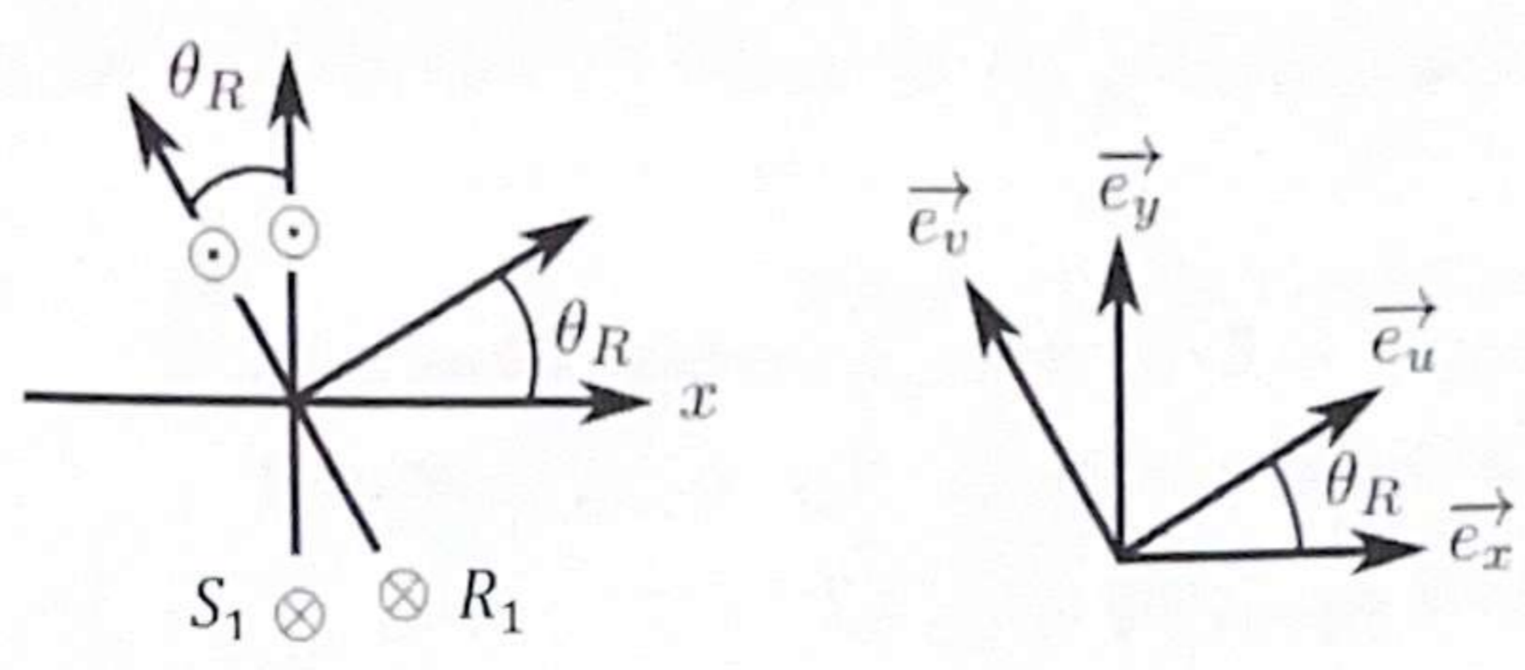
Figure 12 - Repérage de la position \theta_R du rotor
