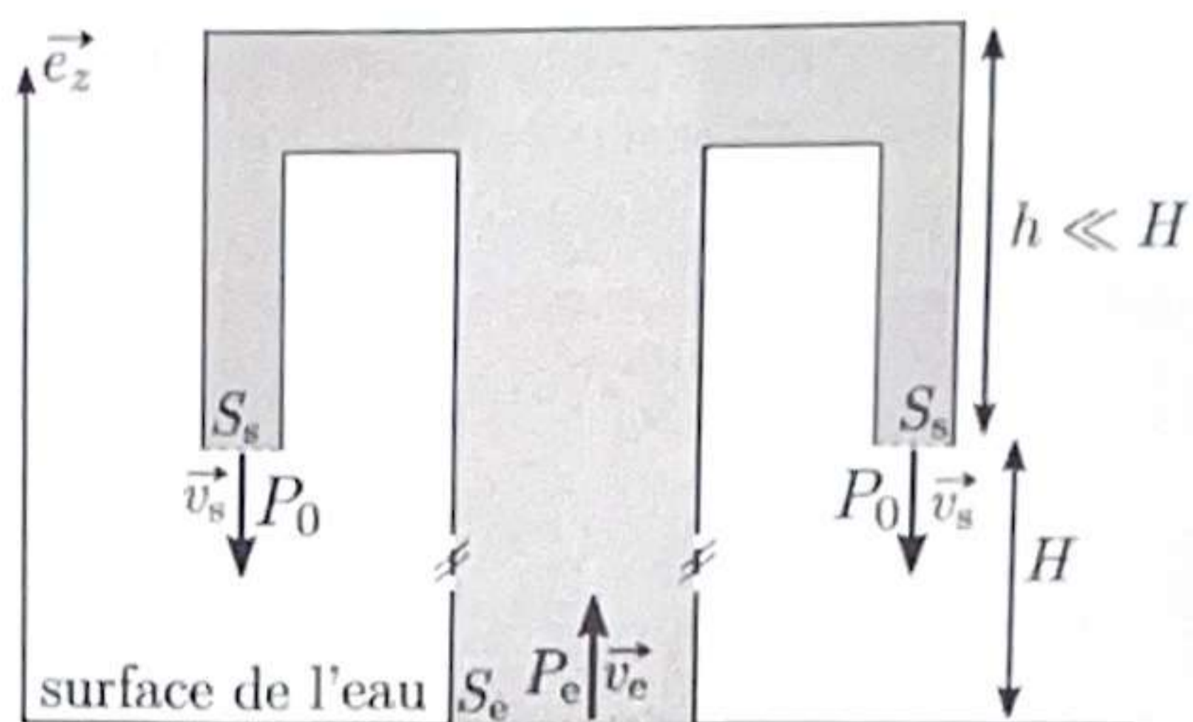
Figure 2 - Schématisation du flyboard
