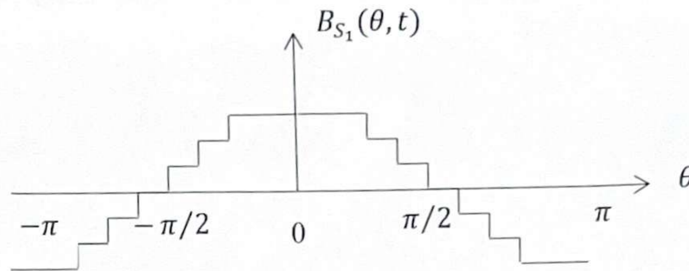
Figure 11 - Modélisation simplifiée du champ créé par l'ensemble des spires de l'enroulement S_1 dans l'entrefer
