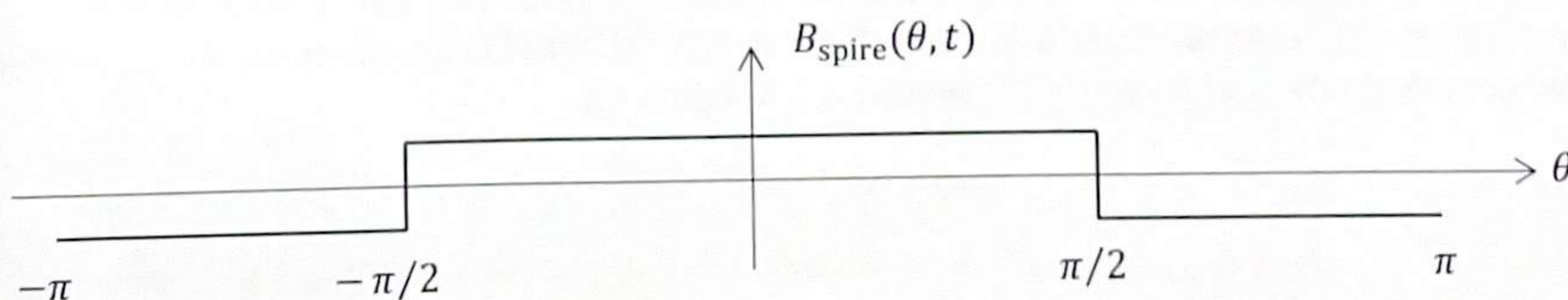
Figure 10 - Modélisation simplifiée du champ créé par une seule spire de S_1 dans l'entrefer
