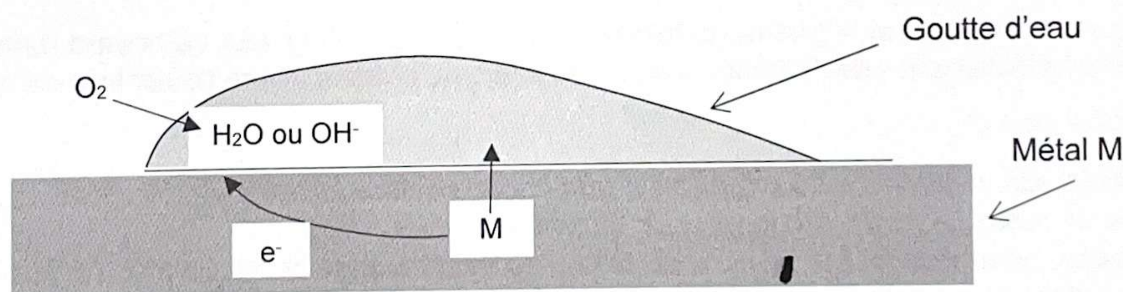
Figure 4 - Corrosion d'un métal par une goutte d'eau
