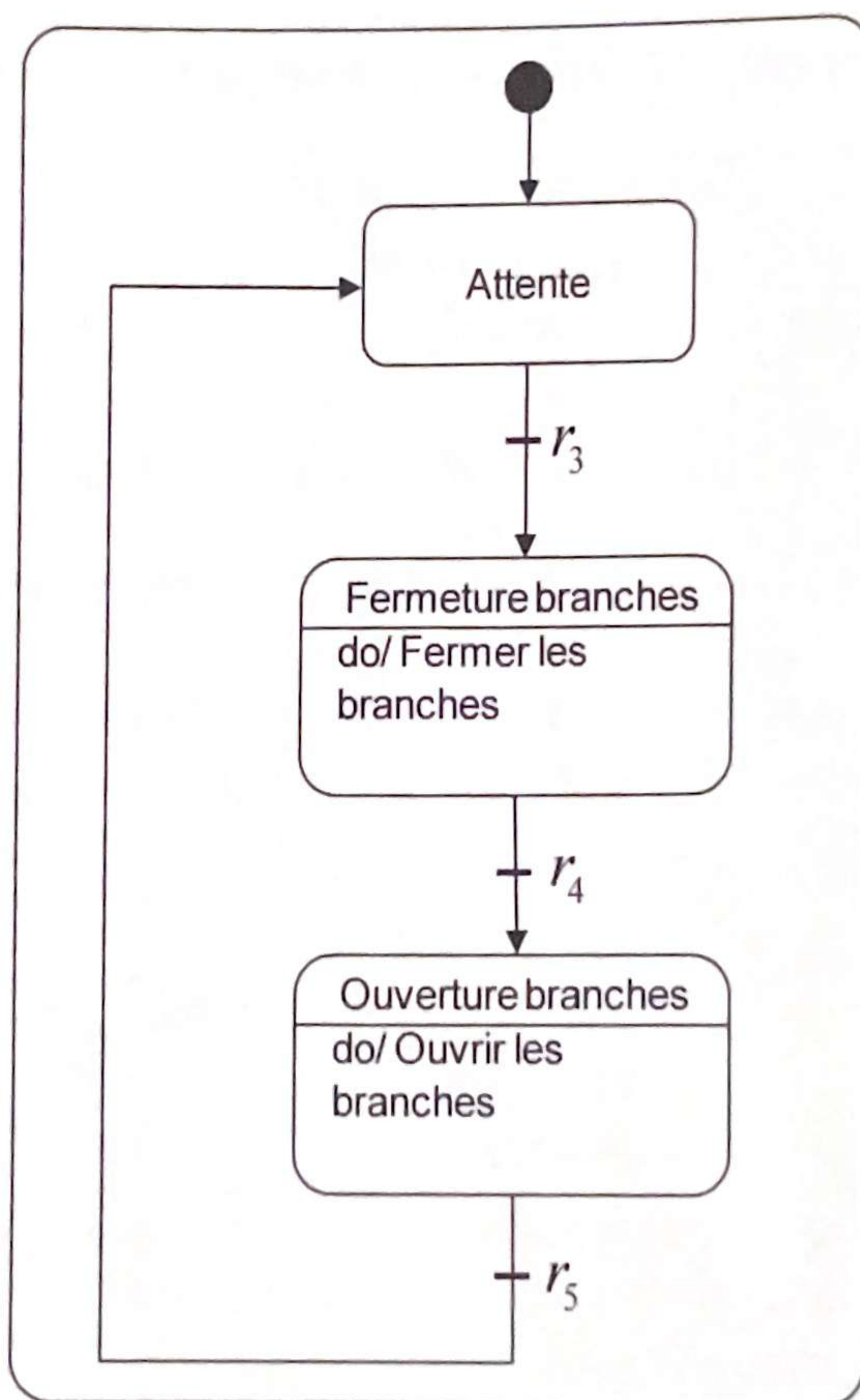
Figure 17 - Diagramme d'état pour simulation d'une pince brucelles inversée
