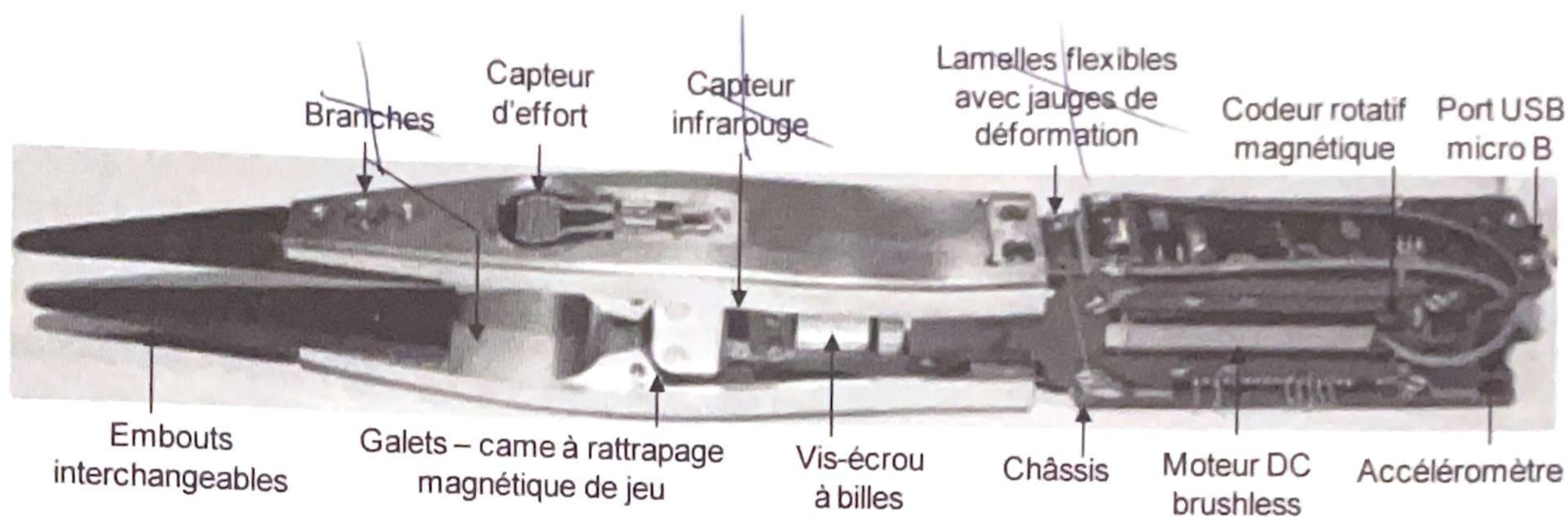
Figure 3 - Pince instrumentée – vue détaillée
