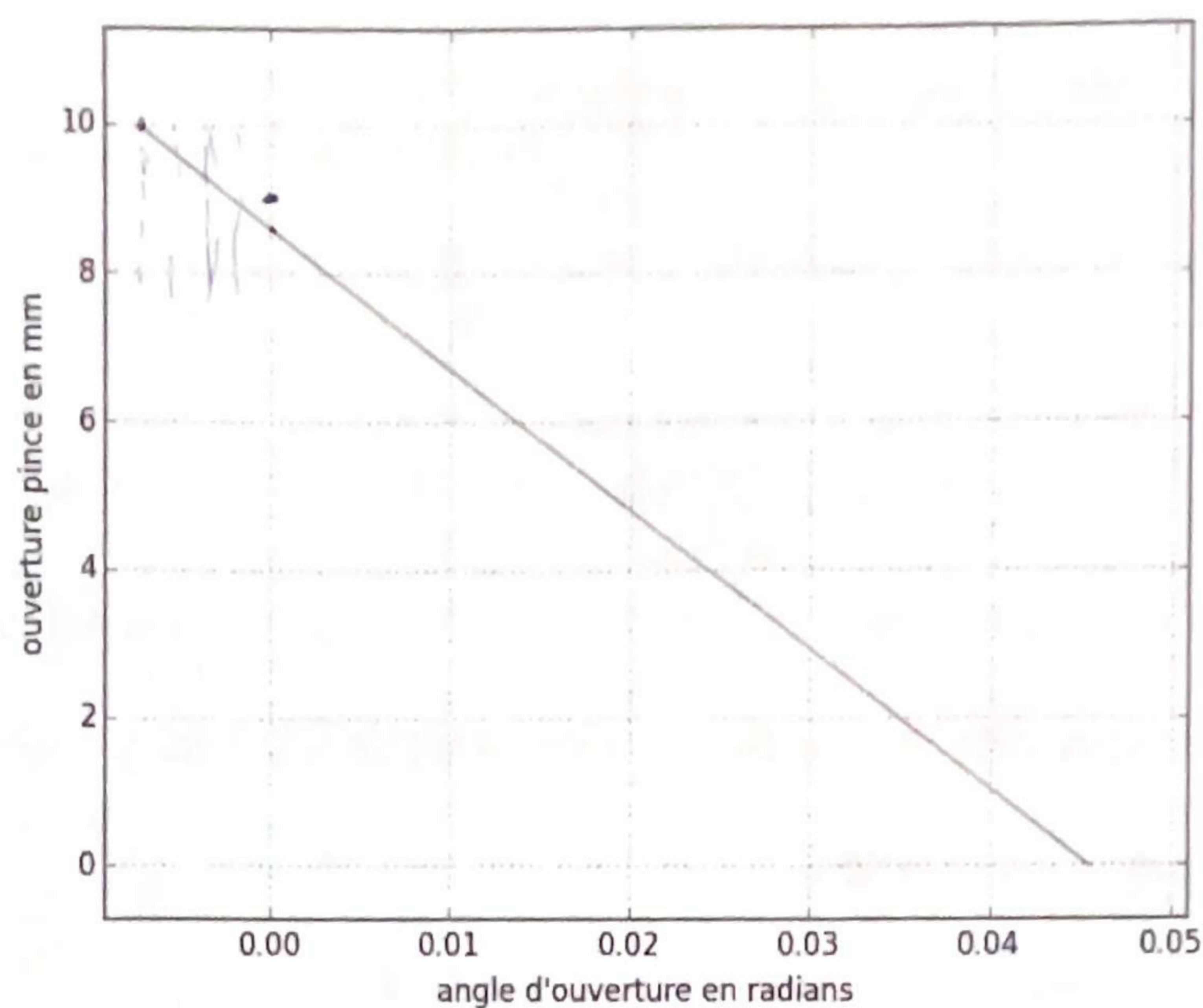
Figure 4 - Ouverture de la pince en fonction de l'angle d'ouverture \alpha
