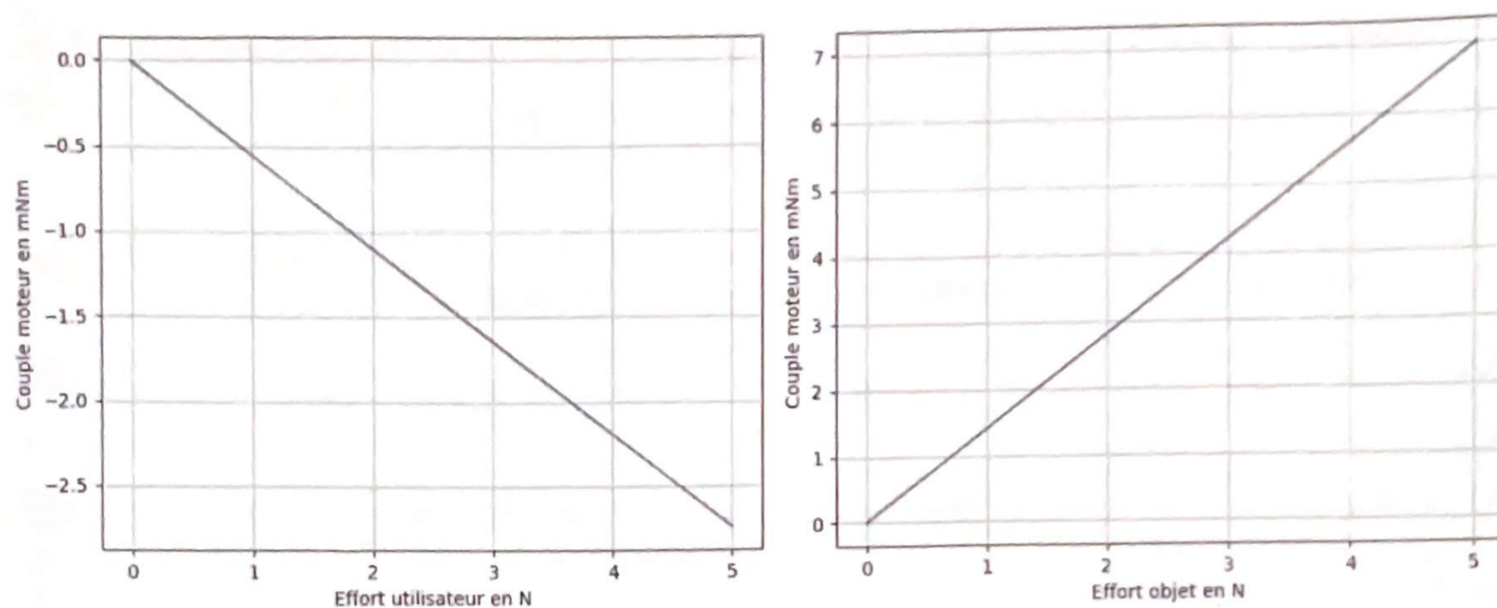
Figure 6 - Couple moteur en fonction de l'effort de l'utilisateur (gauche) ou de l'objet (droite)
