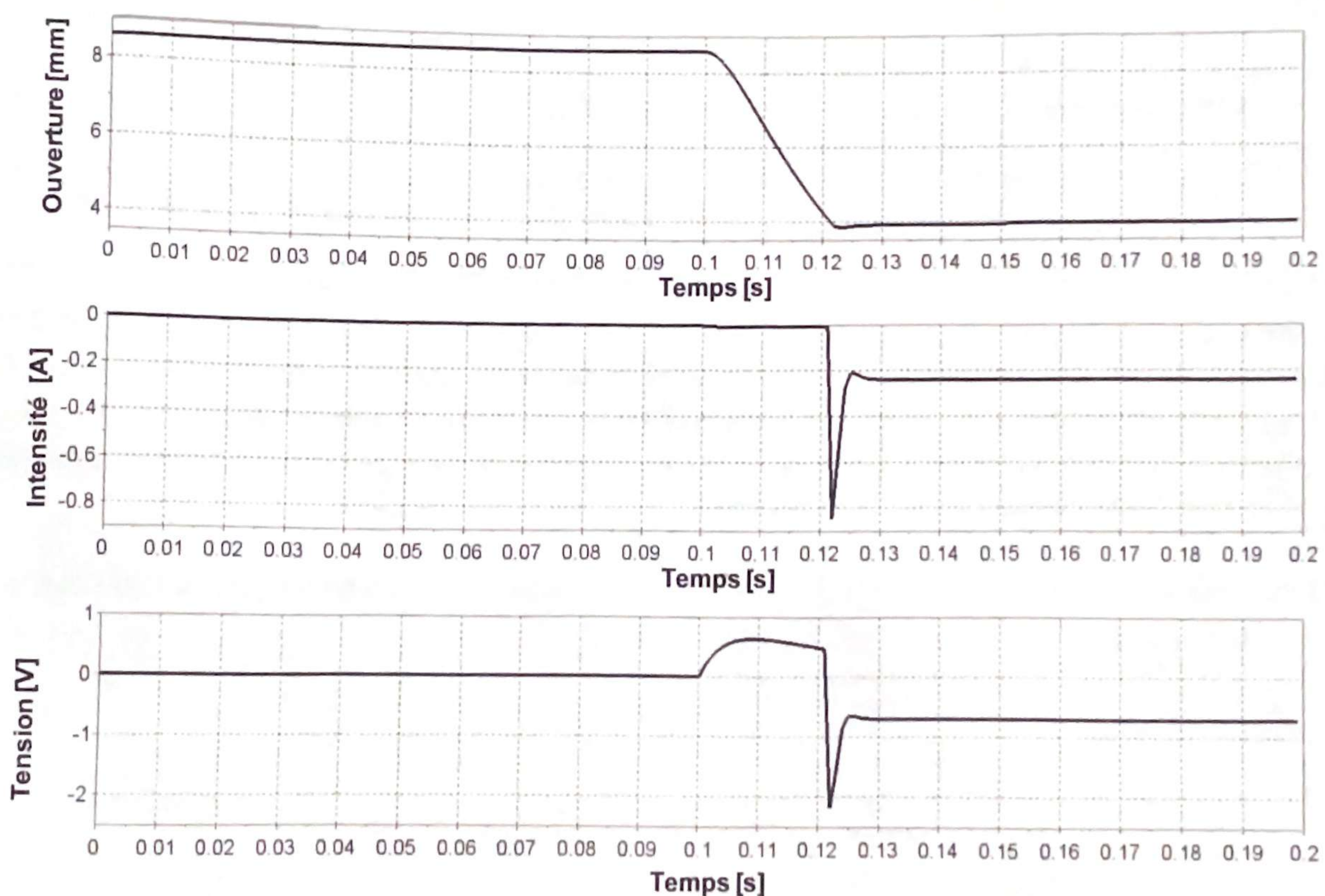
Figure 8 - Réponses temporelles d'ouverture, d'intensité et de tension pour un objet simulé de taille 4 mm suite à une action de l'utilisateur de 3 N à 0,1 s
