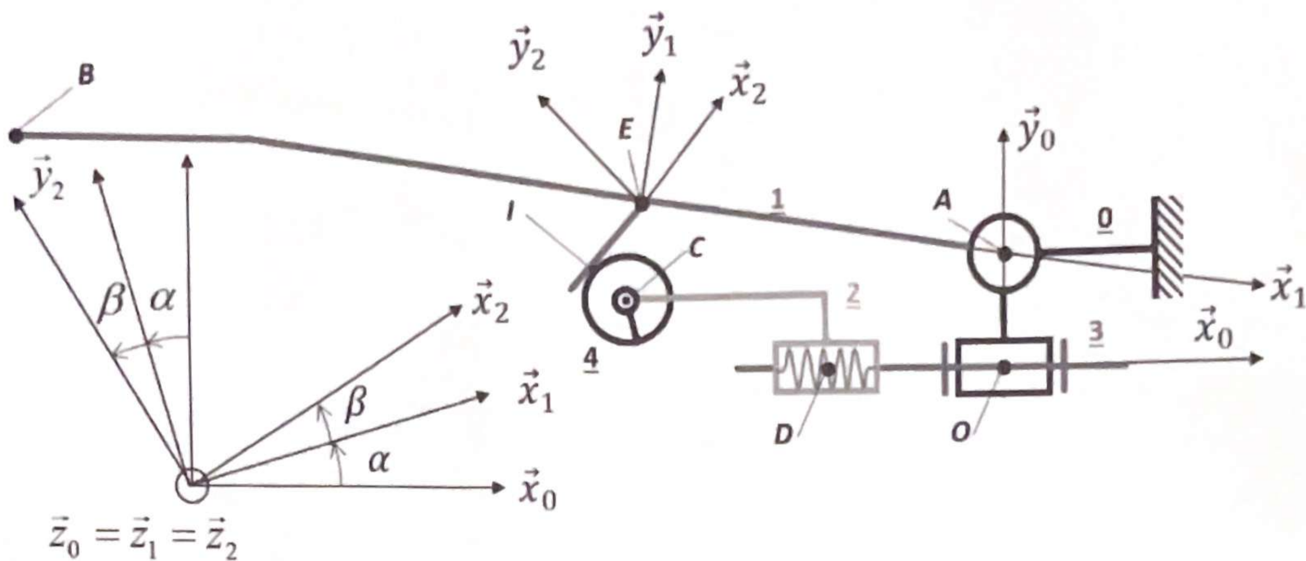
Figure 13 - Modèle géométrique de la demi-pince
