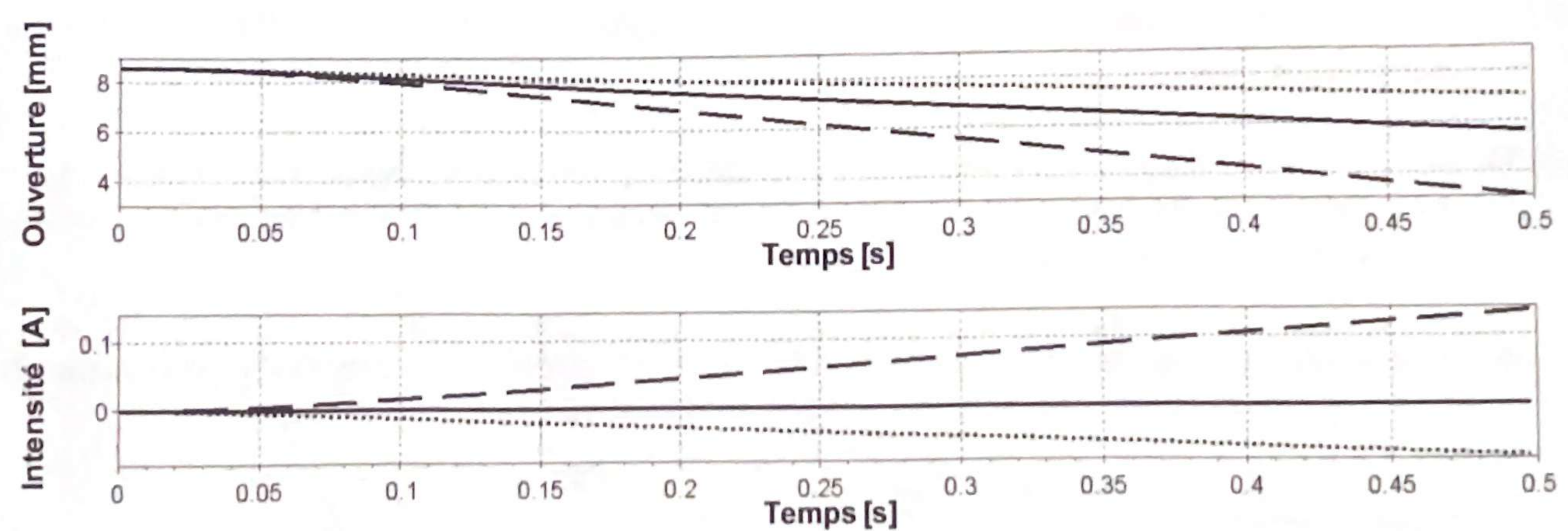
Figure 7 - Réponses temporelles d'ouverture et d'intensité suite à une action de l'utilisateur de type rampe de pente 2 N/s pour des raideurs souhaitées C_a
