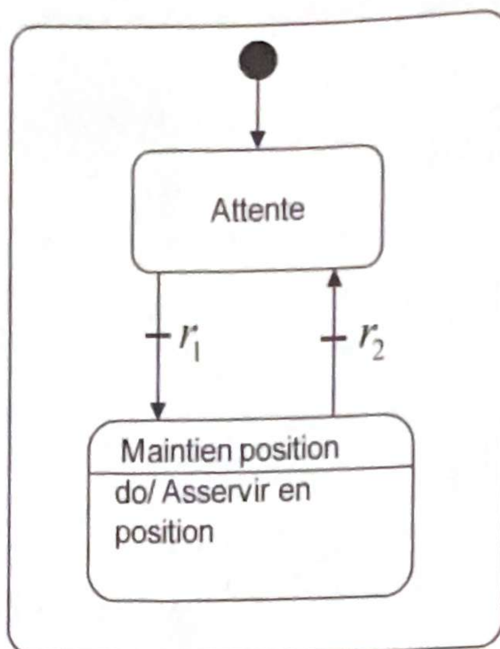
Figure 16 - Diagramme d'état pour blocage de la fermeture
