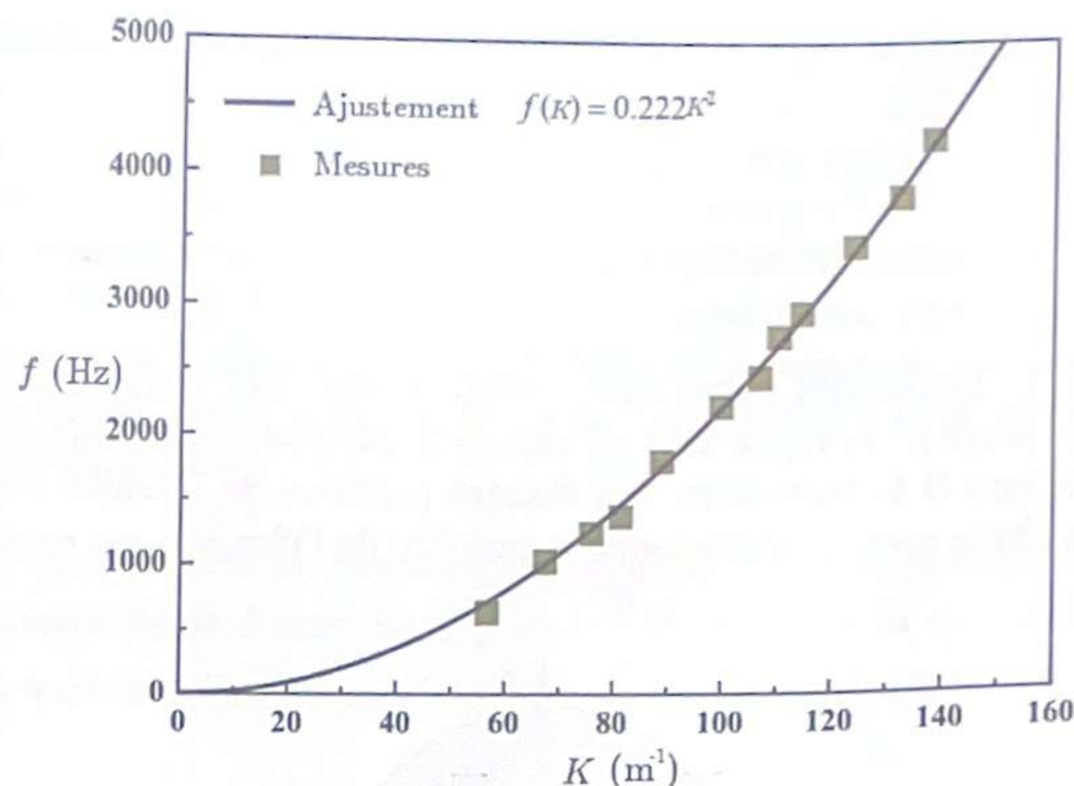
FIGURE 6 – Évolution de la fréquence f_i des modes de résonance en fonction du nombre d'onde K_i . L'ajustement en traits pleins a pour équation f(K) = 0,222 K^2 . Source : The Journal of the Acoustical Society of America 137 (2015).
