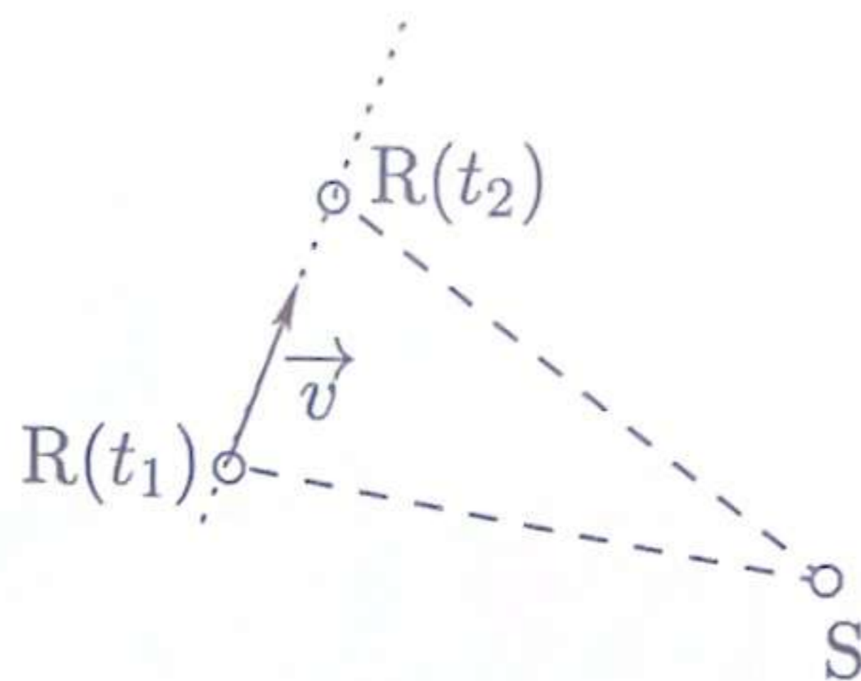
FIGURE 8 – Modélisation de l'effet Doppler lorsque le récepteur est en mouvement par rapport à la source, supposée immobile.
