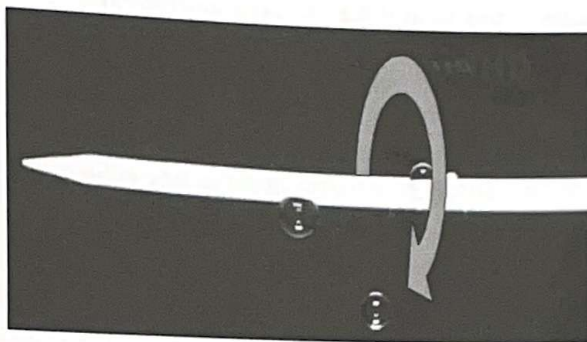
FIGURE 1 – Expérience de D. Pettit. La flèche grisée indique une rotation de la goutte autour de l'axe de l'aiguille.
