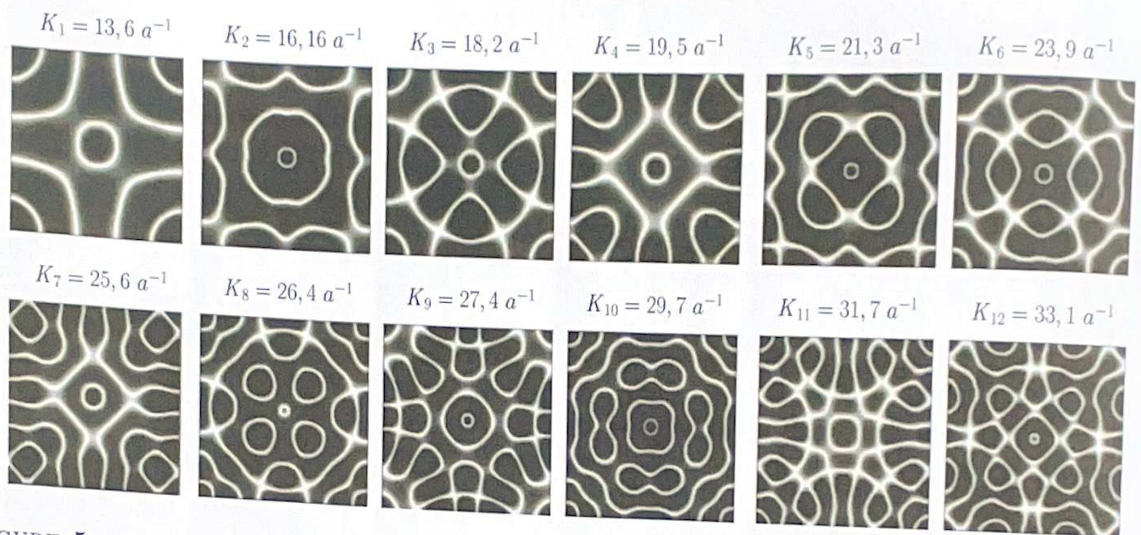
FIGURE 5 – Valeurs de K_i correspondant aux modes associés aux figures de Chladni illustrées sur la figure 4. Les motifs représentés sur la figure sont issus de simulations numériques. Source : The Journal of the Acoustical Society of America 137 (2015).
