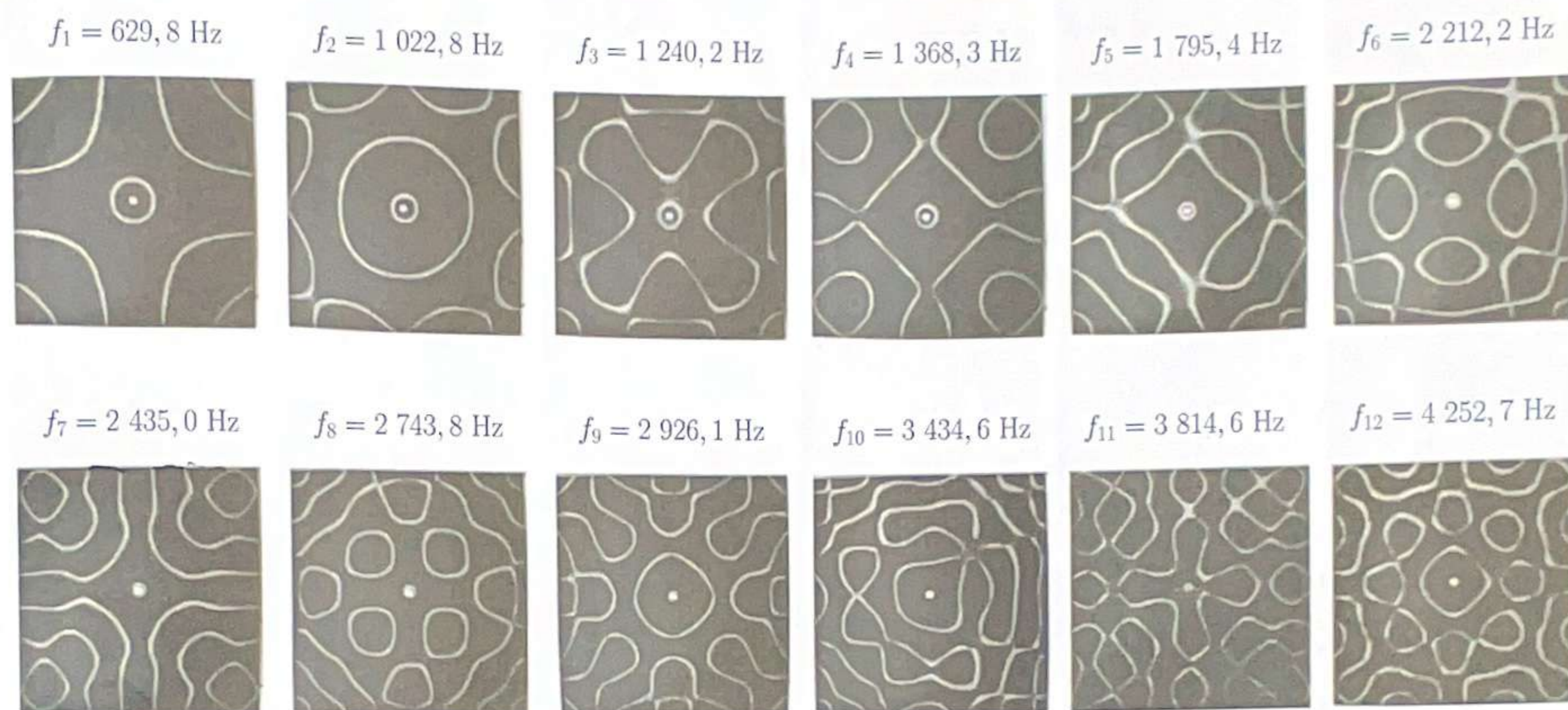
FIGURE 4 – Figures de Chladni observées avec la plaque d'épaisseur h_1 = 1 mm. Pour chaque mode de résonance (un motif spatial), on précise la fréquence f_i associée, avec i = 1, \dots, 12 . Source : The Journal of the Acoustical Society of America 137 (2015).
