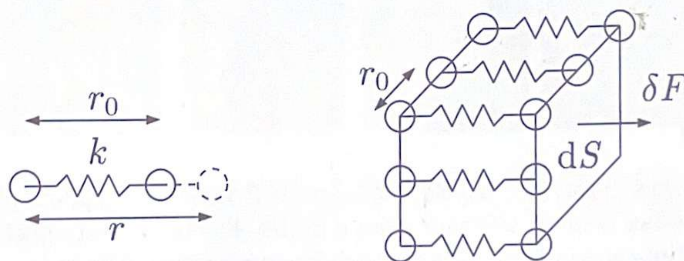
FIGURE 2 – Modélisation microscopique des liaisons entre atomes dans un réseau cubique.
