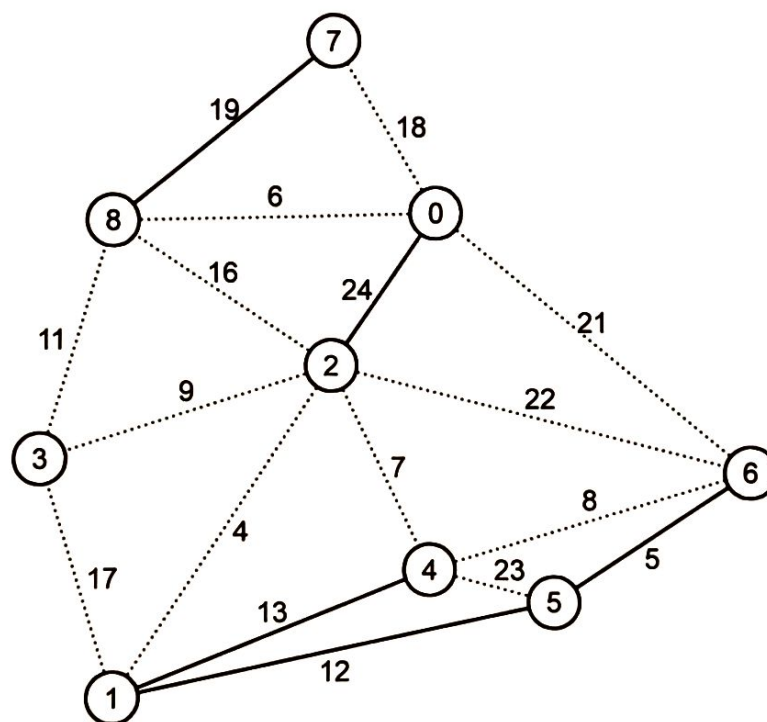
Figure 4 - Un sous-graphe H du graphe de la figure 2 , comportant quatre composantes connexes. Les arêtes qui n'appartiennent pas au sous-graphe sont représentées en pointillés
