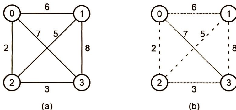
Figure 5 - (a) Le graphe correspondant au réseau de l'île de Korfe. (b) Exemple de configuration finale (contrôlée par MaxDébit) atteinte à l'issue d'une partie. Les arêtes choisies par le joueur MaxDébit sont représentées par un trait discontinu et celle par le joueur MinLatence par une ligne en pointillés
