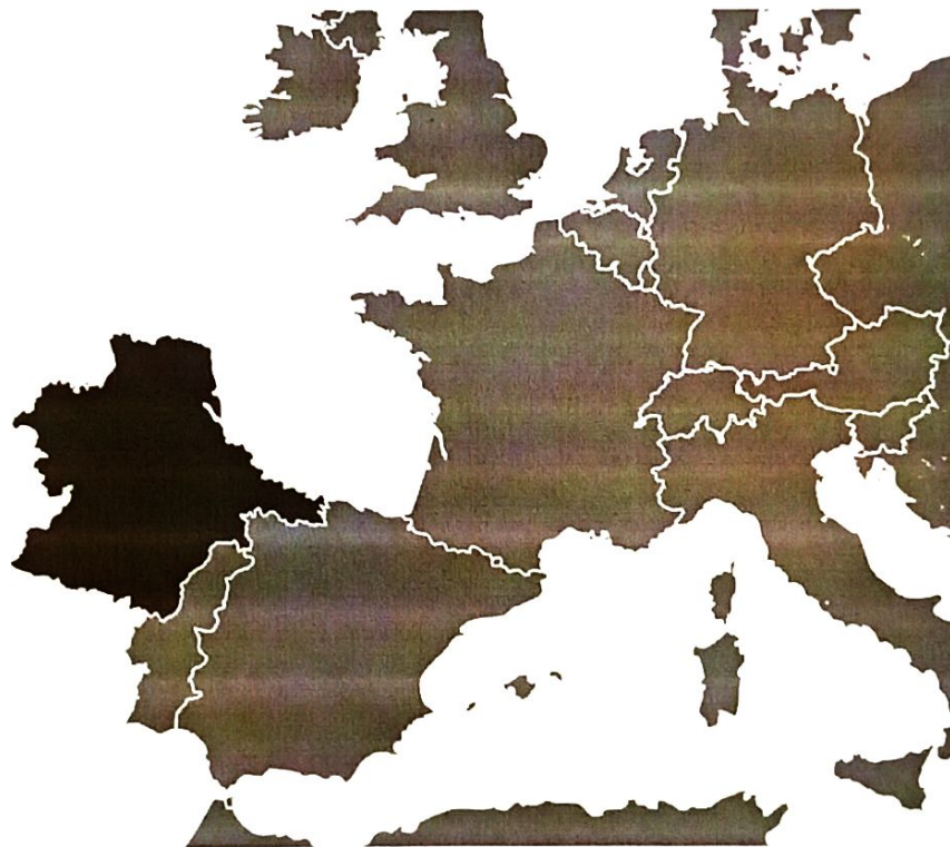
Figure 1 - La république imaginaire du Listenbourg
