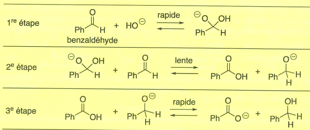
Schéma 7 - Réaction de Cannizzaro avec le benzaldéhyde (Ph = phényle = -\text{C}_6\text{H}_5 )
