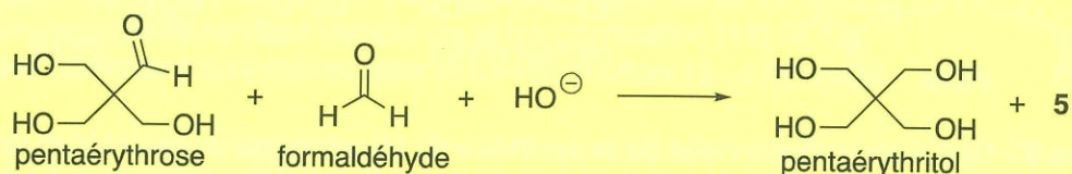
Schéma 6 - Réaction de Cannizzaro croisée entre le pentaérythrose et le formaldéhyde
