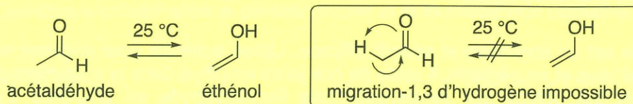
Schéma 1 - Équilibre tautomérique céto-énolique de l'acétaldéhyde
