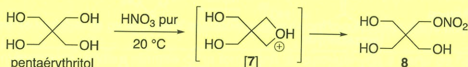
Schéma 9 - Séquence réactionnelle de la première étape de la synthèse du tétranitrate de pentaérythritol
