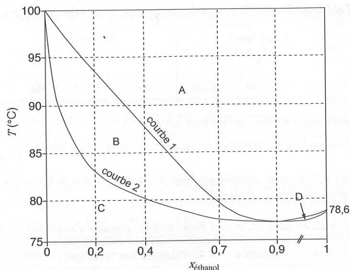
Figure 2. Diagramme binaire isobare liquide-vapeur du mélange eau-éthanol ( P = 1 bar).
