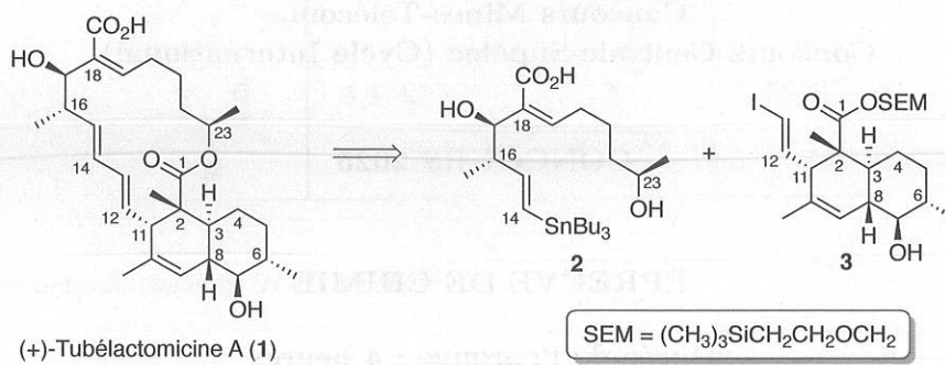
Schéma 1. Approche rétrosynthétique de la (+)-tubélastomine A.
