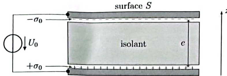
FIGURE 6 – Hygromètre capacitif en l'absence d'humidité
