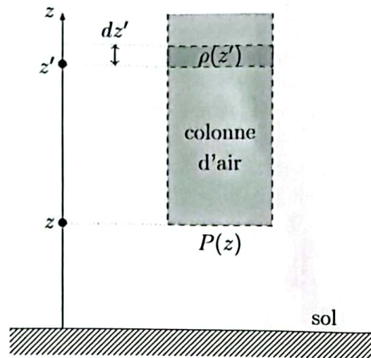
FIGURE 1 – Équilibre d'une colonne d'air
