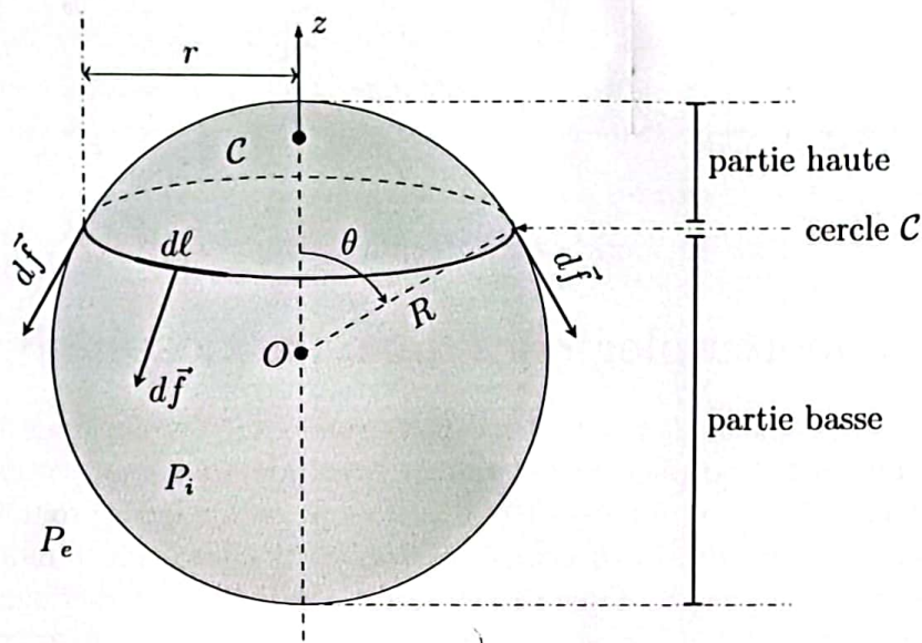
FIGURE 3 – Forces de tension au sein de la membrane du ballon
